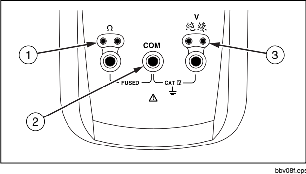
图 4. 输入端子
