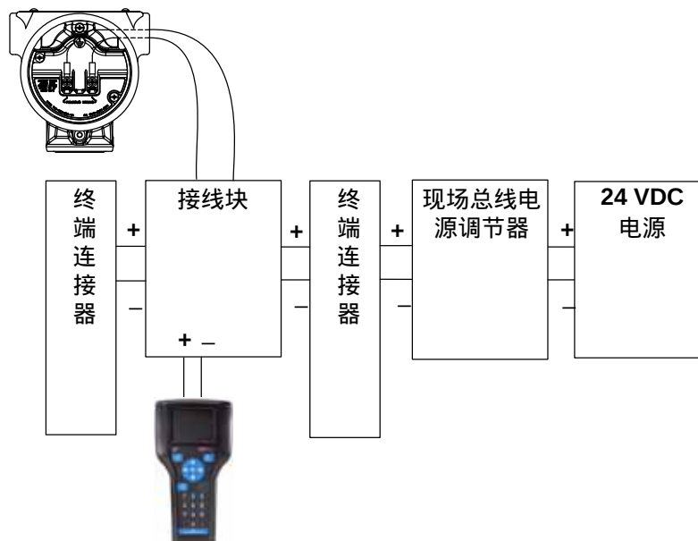
图 4-3. 工作台接线图示例
