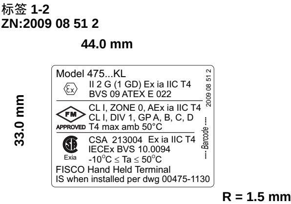
图 B-2. Ex 认证标签示例（仅在具有 KL 选项的 475 现场通讯器上。）
