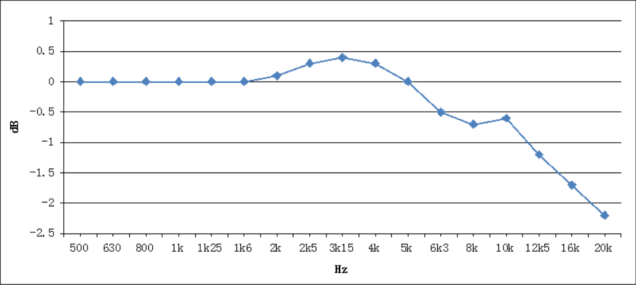
指向设为 90 时的 Z 计权响应
