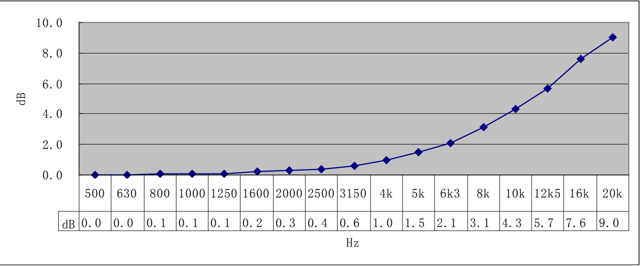
指向设为 90 时的 Z 计权响应
