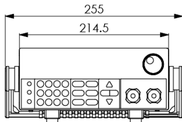
详细尺寸图
