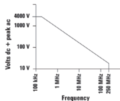
10076B 降额曲线
