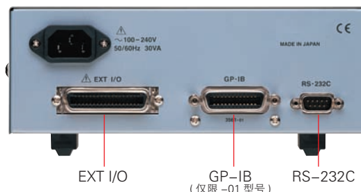
3561-01 背面
