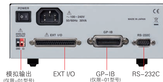
BT3563-01、BT3562-01 背面
