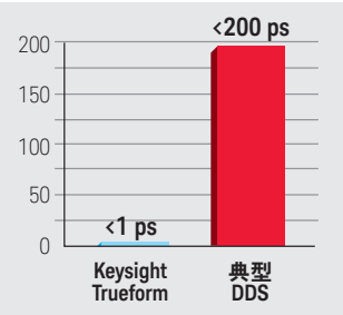
抖动
