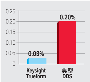
总谐波失真
