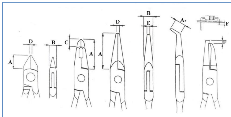
Head Types 剪钳头部种类
