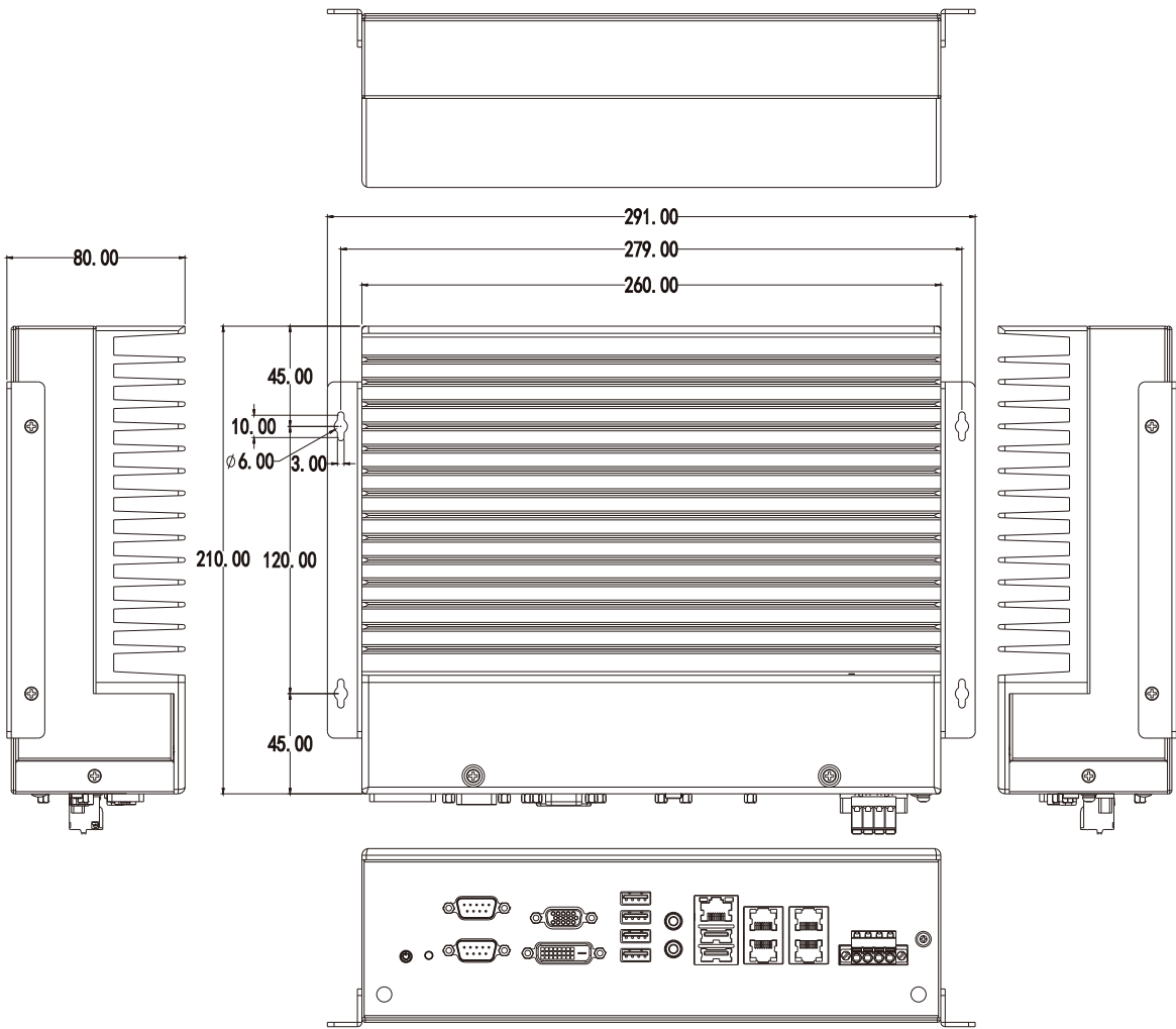
结构图
