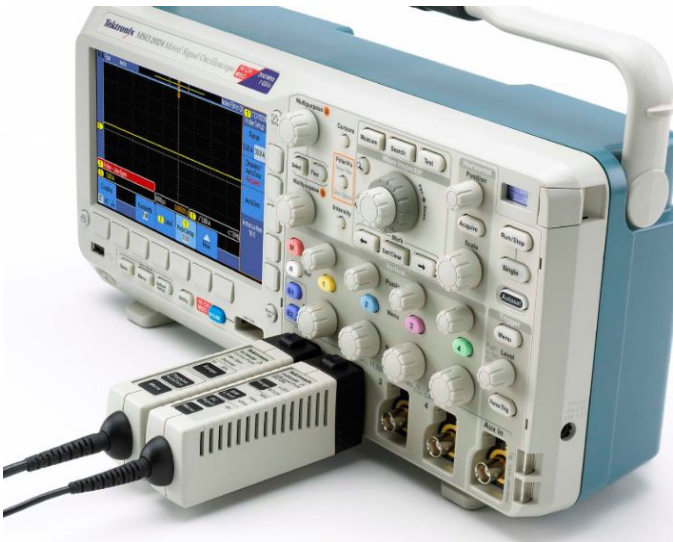
TekVPI 探头接口简化探头与示波器的连接。
