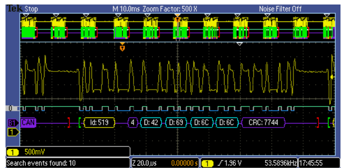
搜索步骤 2：Wave Inspector 自动搜索整个记录，并用空心的白色三角形标记处每一个事件。然后，可以使用 Previous（上一个）和 Next（下一个）按钮在事件之间切换。
