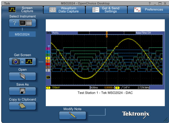
OpenChoice® Desktop 软件实现示波器与 PC 之间的无缝连接。
