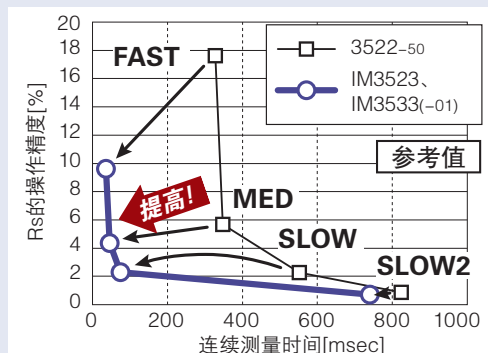
C-D,ESR测量(100kHz)的连续测量时的连续测量时间和Rs的操作精度
