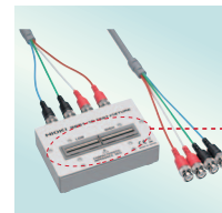
测试治具 9261-10
