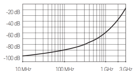
串扰
